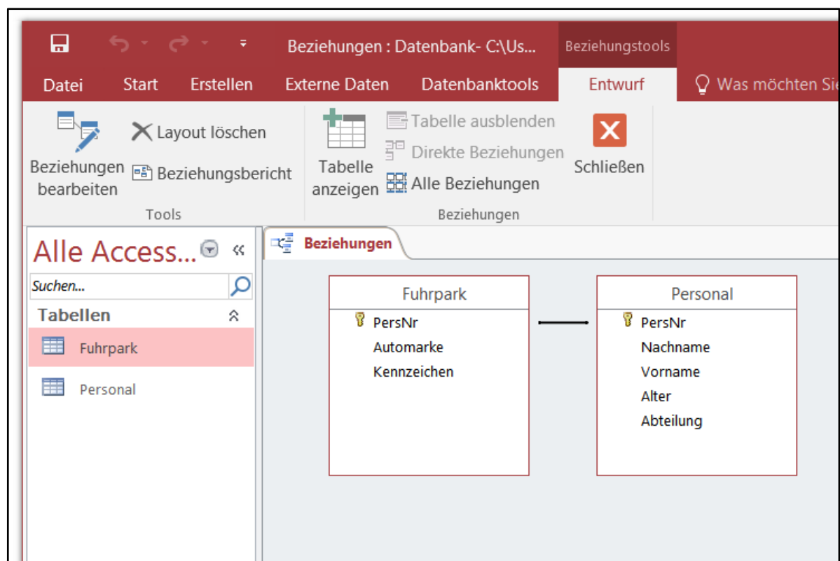
Abb. 169: Beziehung zwischen Tabellen: Lösungsbeispiel 1
