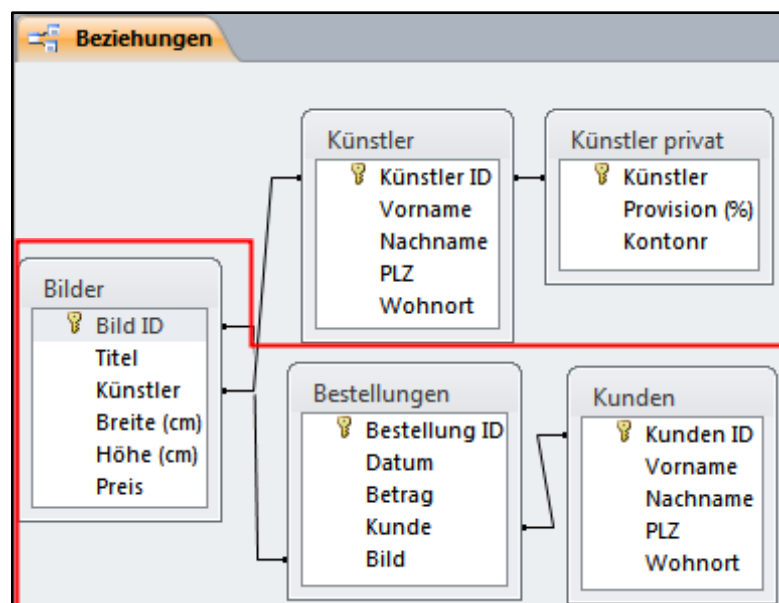
Abb. 168: n:m-Beziehung in Access
