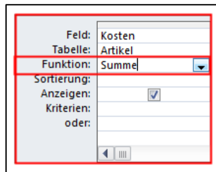
Abb. 182: Funktionen
