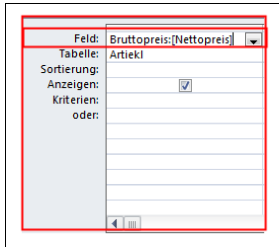
Abb. 184: Neues Datenfeld
