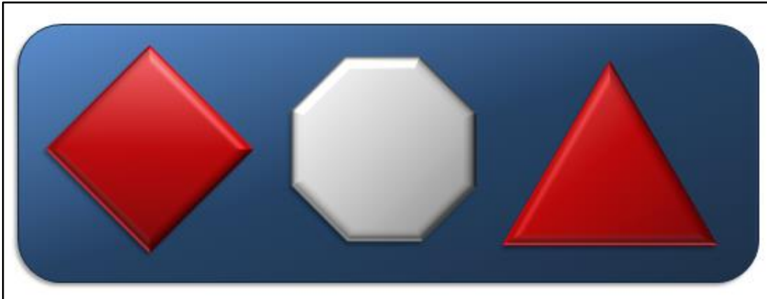
Abb. 173: Beispiel 3
