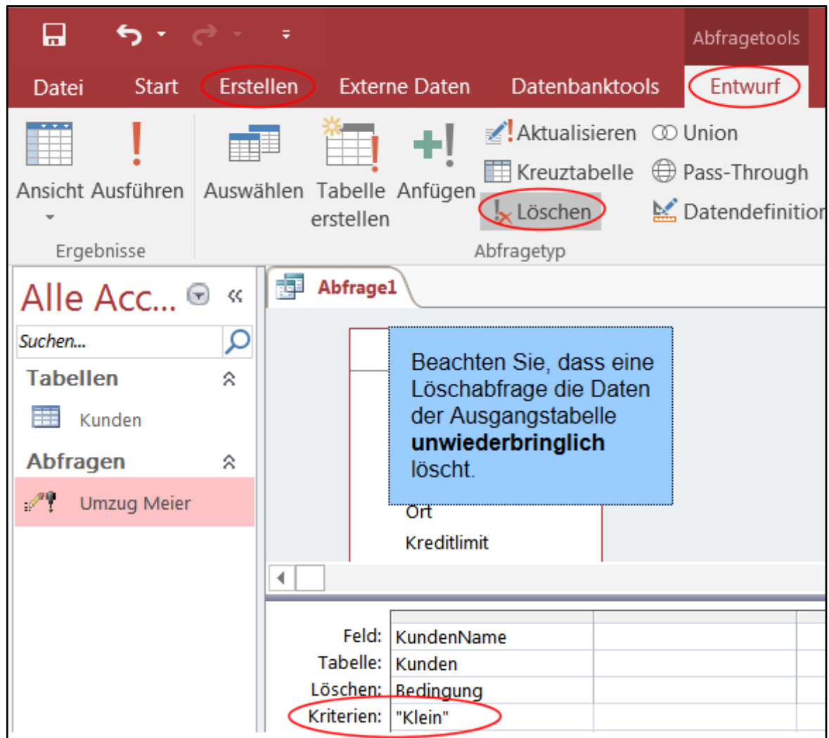
Abb. 191: Löschartfrage
