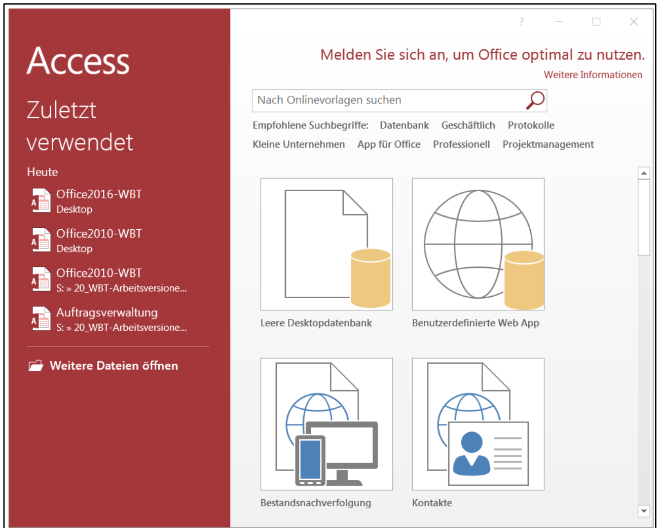
Abb. 145: Access Startbildschirm
