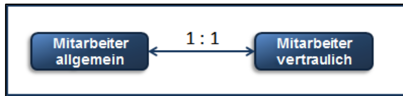
Abb. 165: 1:1-Beziehung
