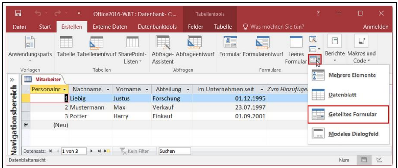
Abb. 159: Geteiltes Formular
