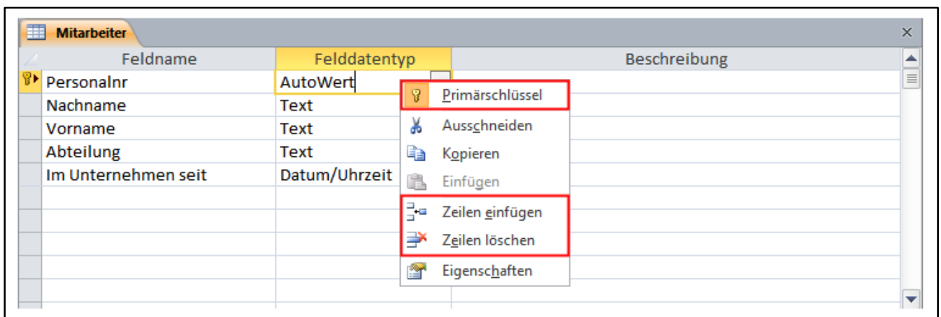
Abb. 155: Entwurfsansicht
