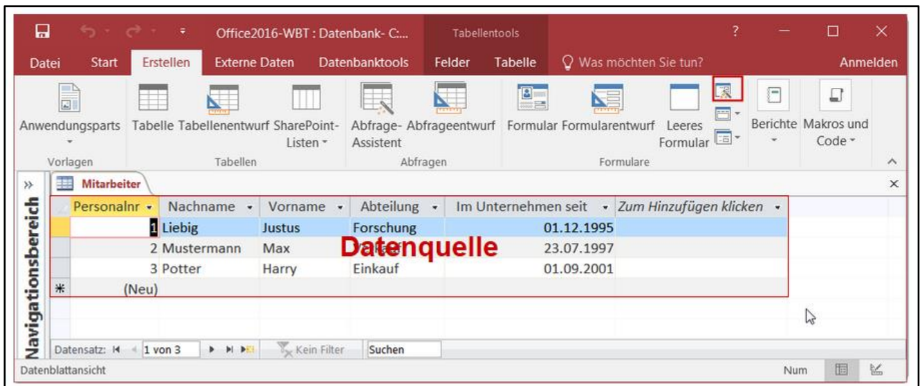
Abb. 162: Formular-Assistent
