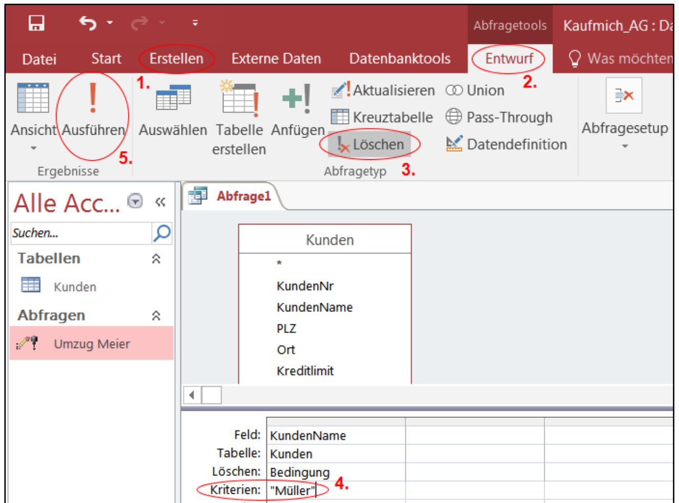
Abb. 192: Lösungsweg Übung Löschabfrage
