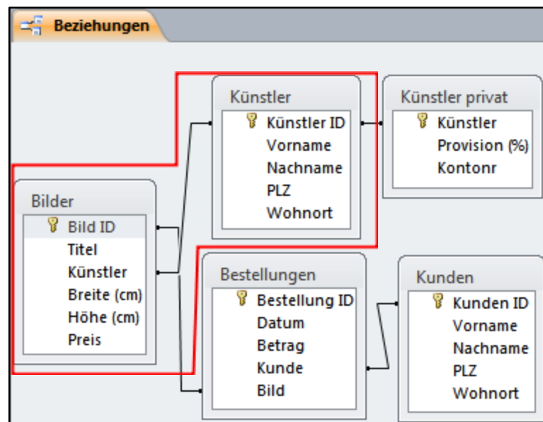
Abb. 164: 1:n-Beziehung in Access
