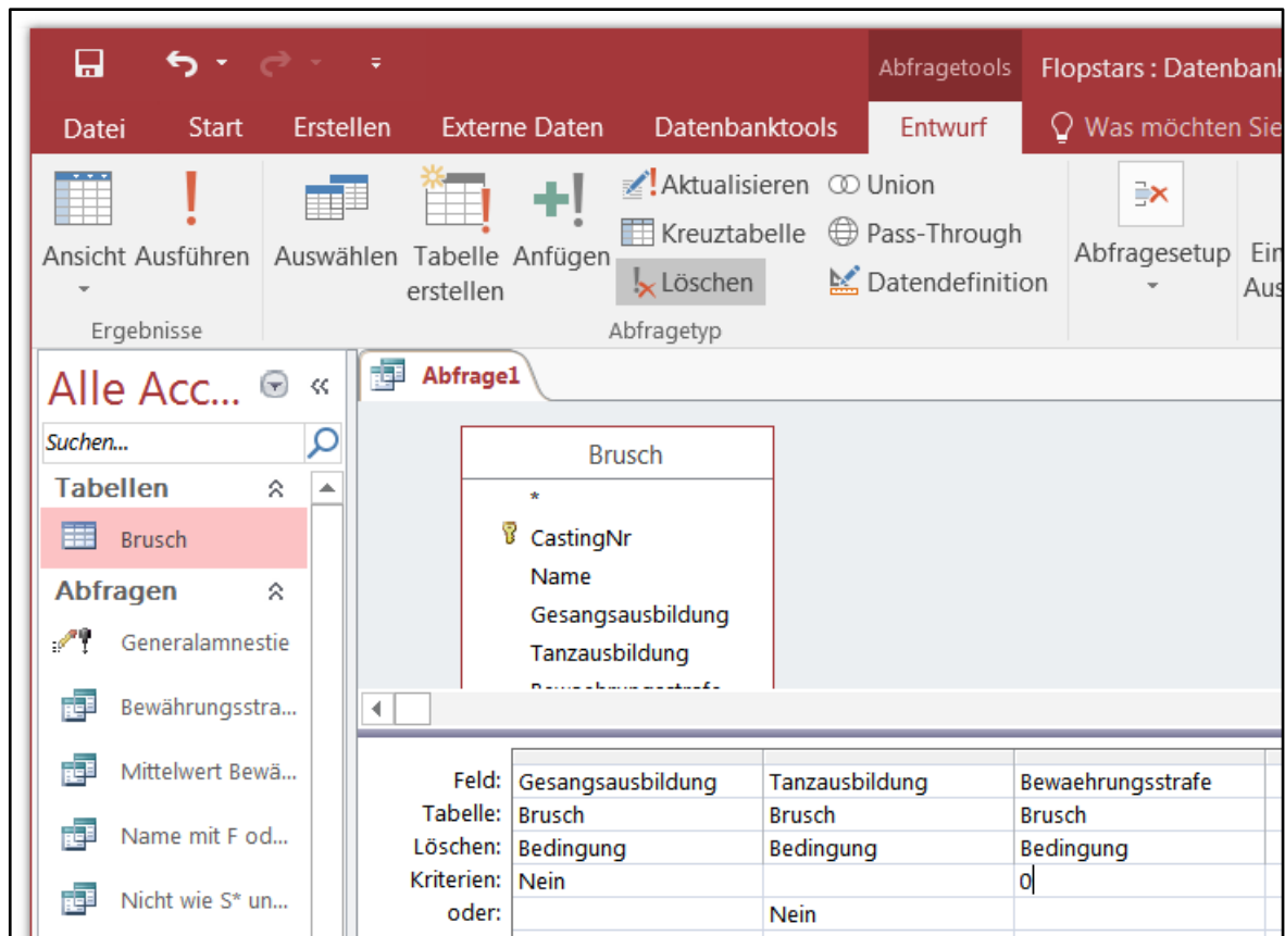
Abb. 206: Lösung 1 zur Übung Flopstars 10
