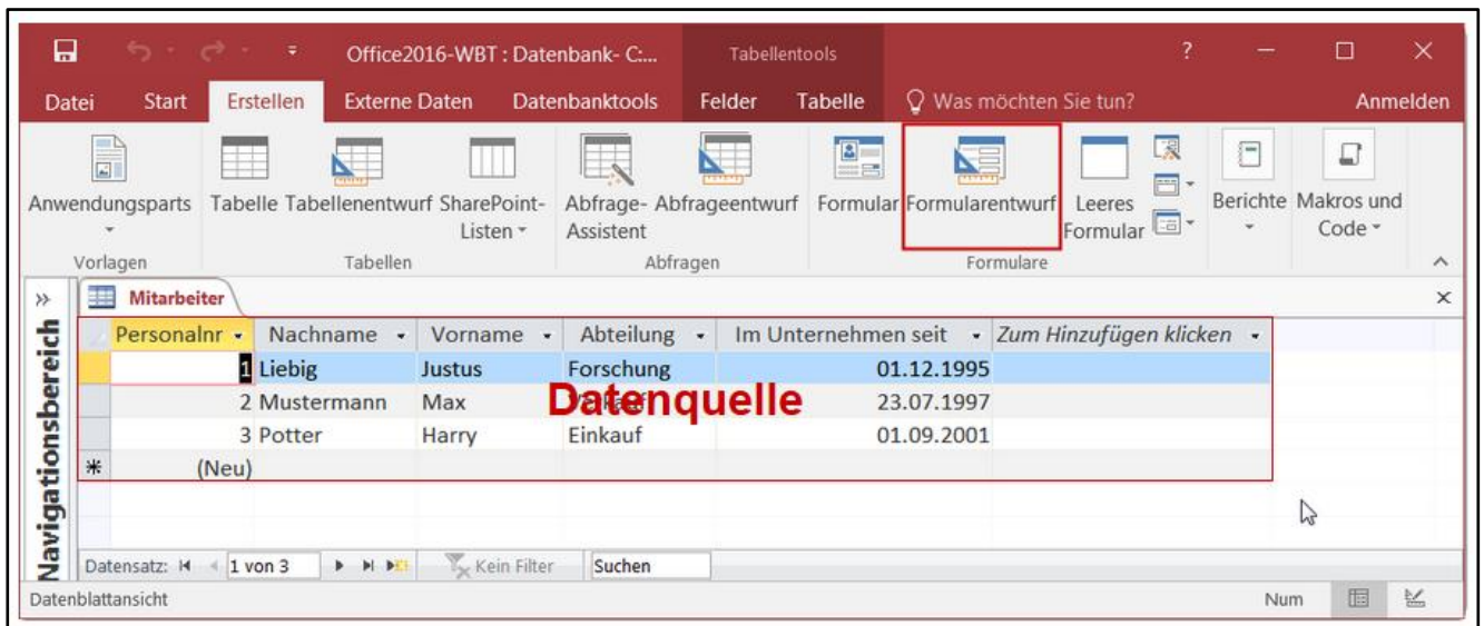
Abb. 161: Formularentwurf
