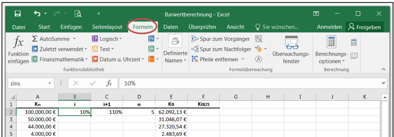
Abb. 65: Funktionsassistent
