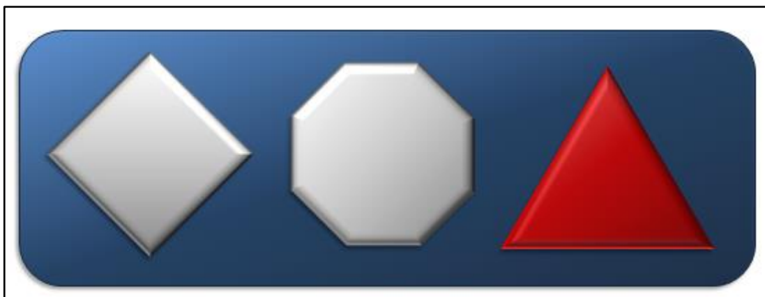
Abb. 172: Beispiel 2
