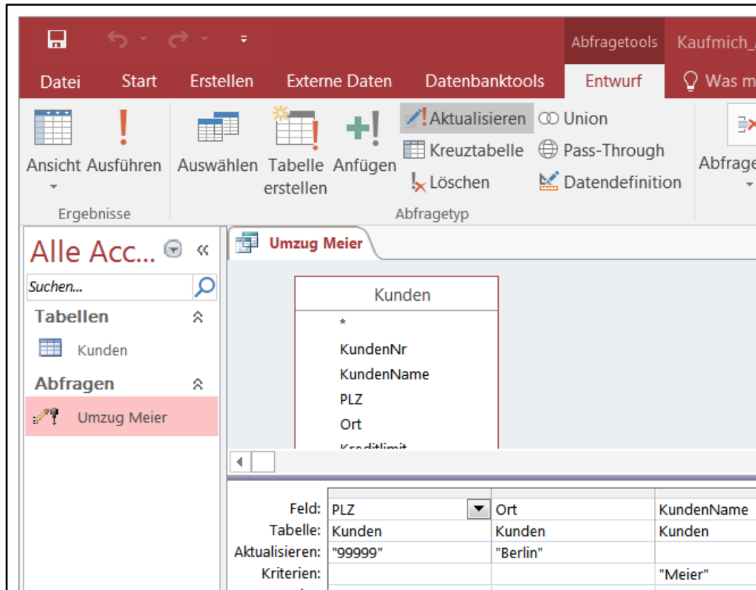
Abb. 190: Übungsaufgabe Aktualisierungsabfrage
