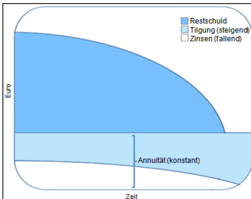
Abb. 118: Annuität
