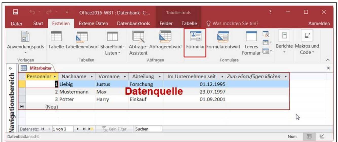
Abb. 158: Einfaches Formular
