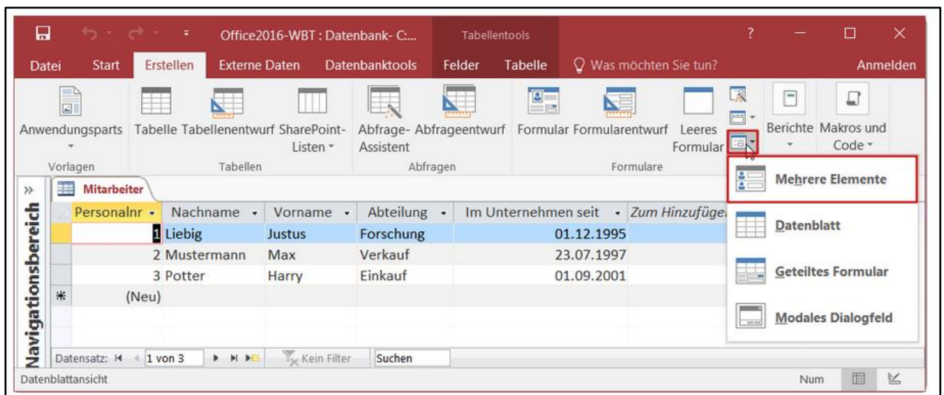
Abb. 160: Mehrere Elemente
