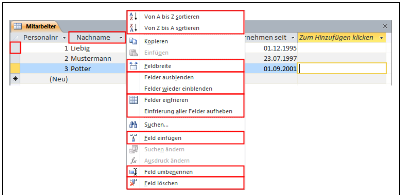
Abb. 157: Datenblattansicht II
