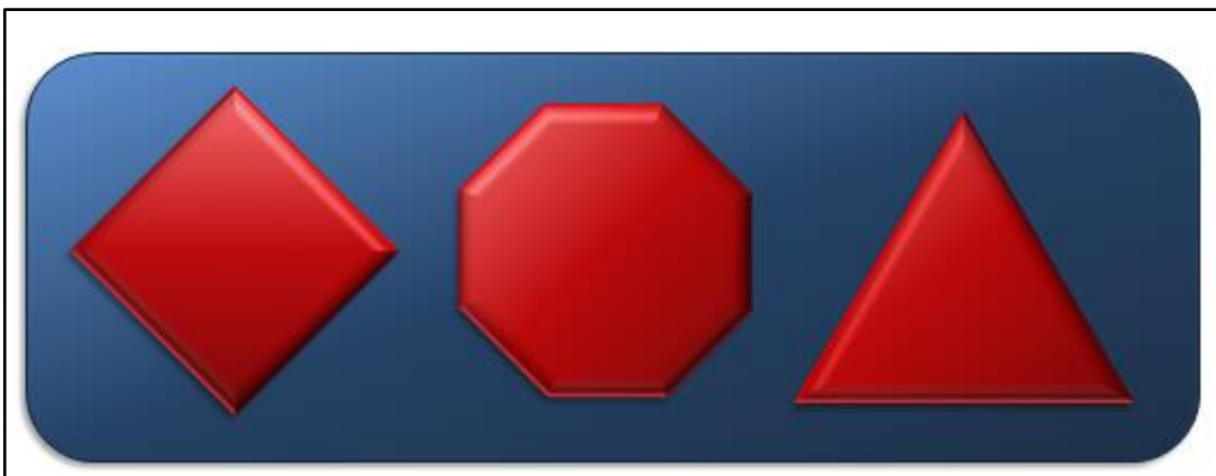
Abb. 175: Beispiel 5
