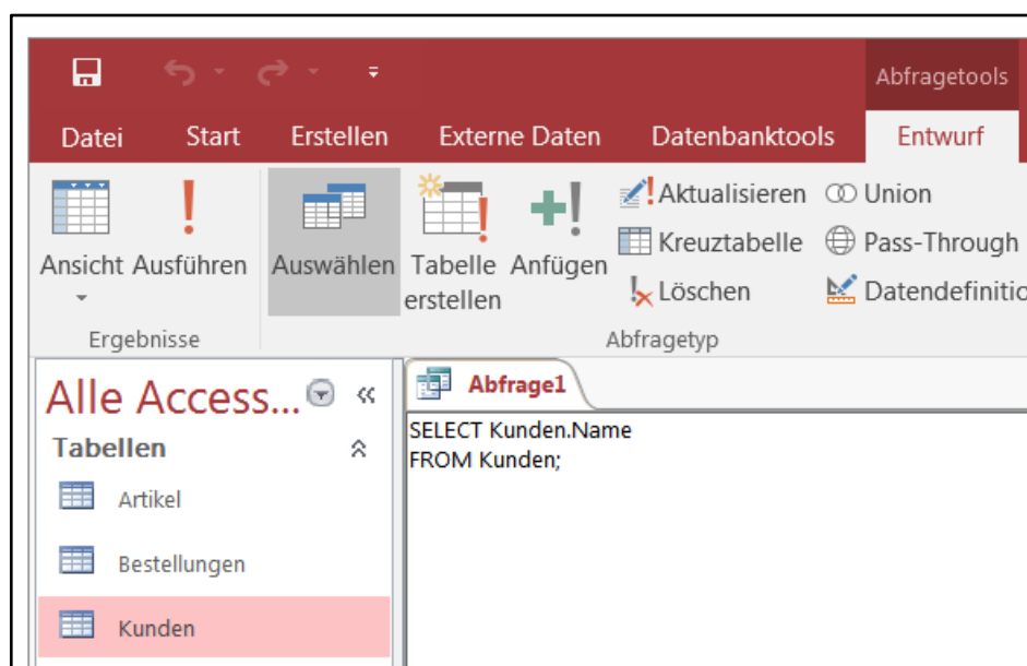
Abb. 209: SQL-Abfrage
