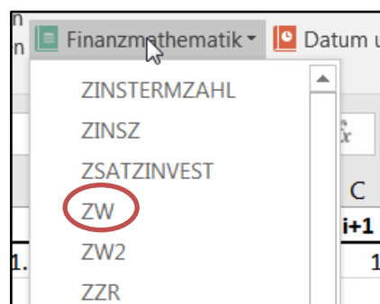
Abb. 69: Funktion ZW
