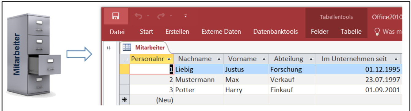
Abb. 141: Veranschaulichung: Datenbanktabellen
