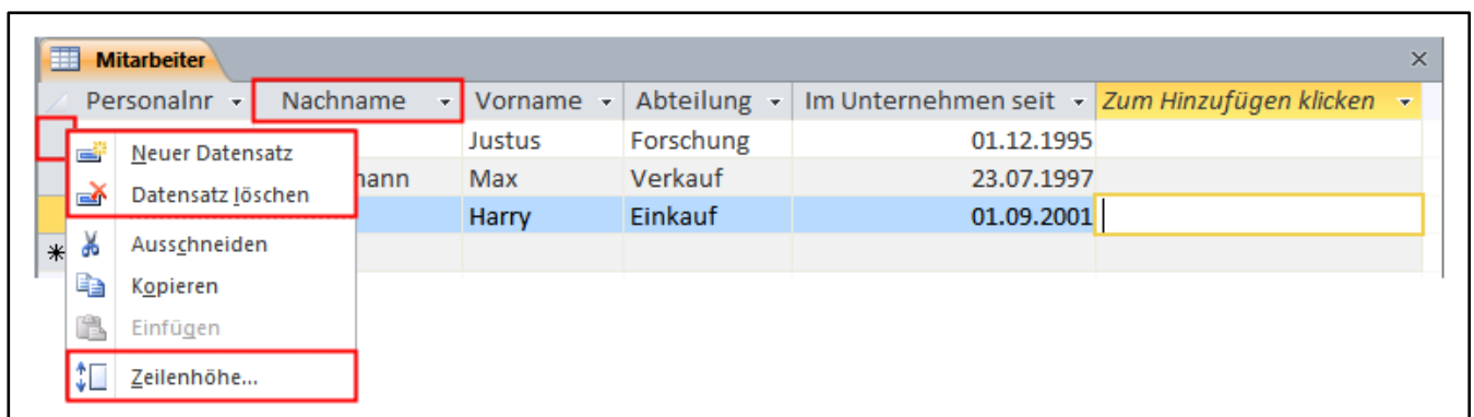
Abb. 156: Datenblattansicht I
