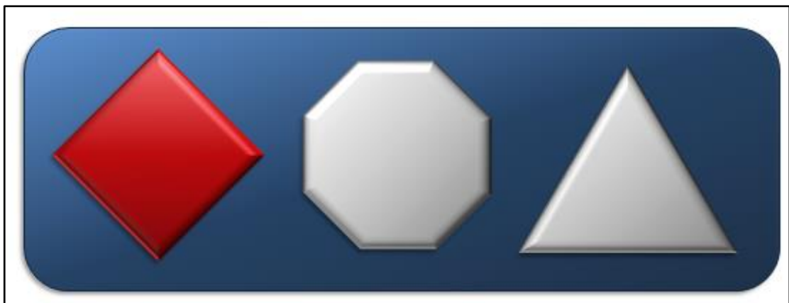
Abb. 171: Beispiel 1
