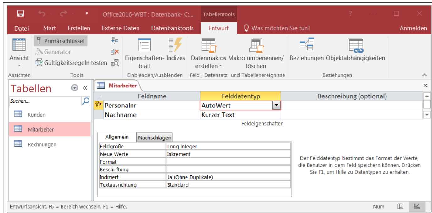
Abb. 154: Entwurfsansicht
