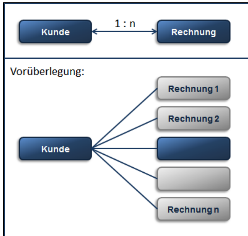
Abb. 163: 1:n-Beziehung
