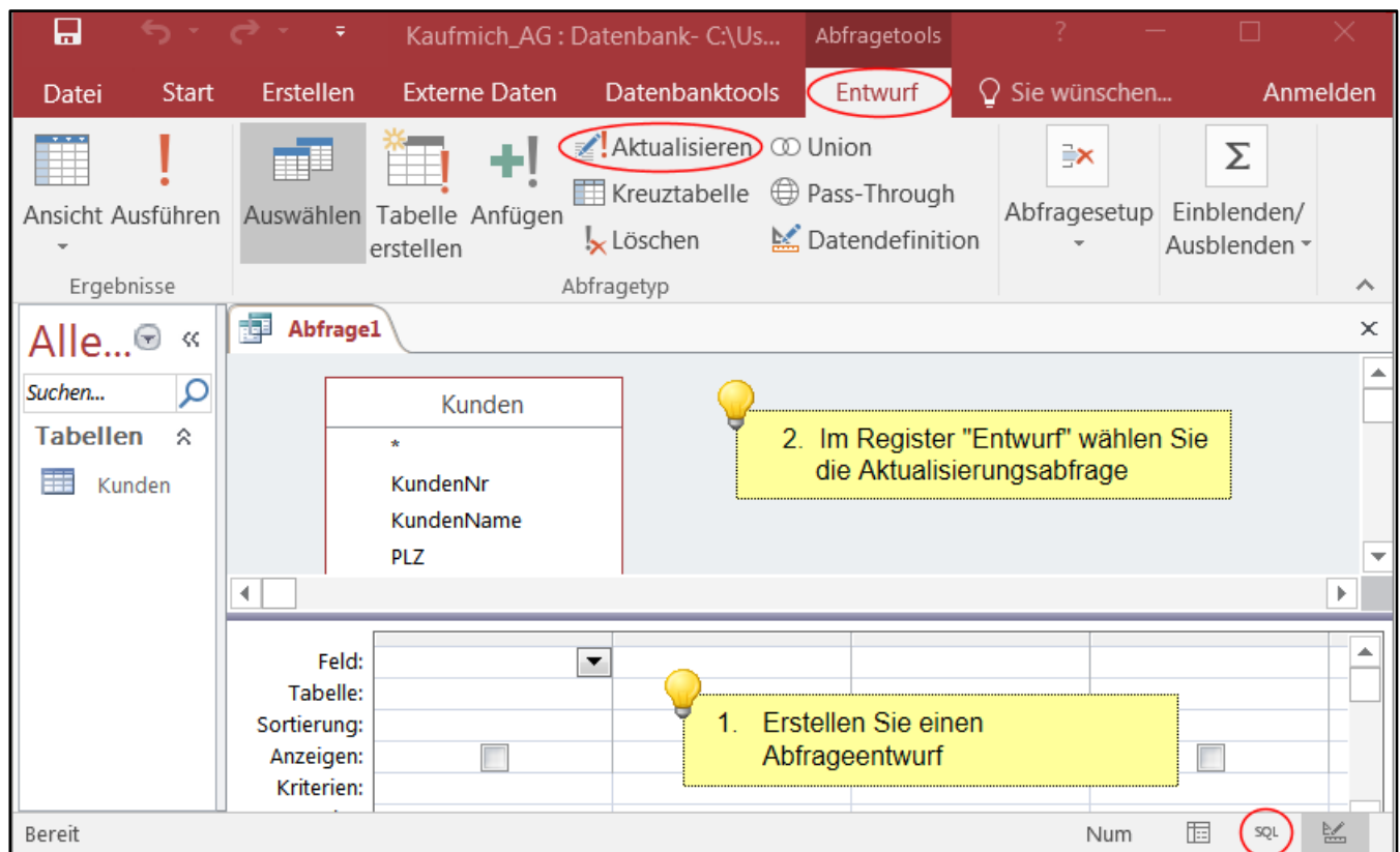
Abb. 188: Aktualisierungsabfrage
