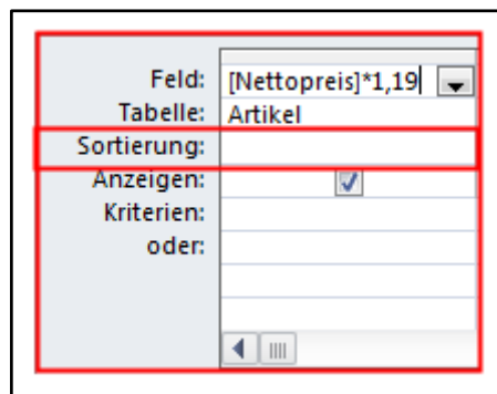
Abb. 183: Operatoren
