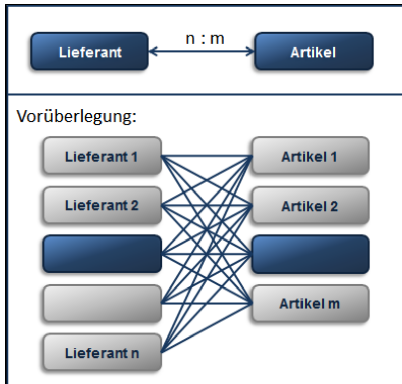
Abb. 167: n:m-Beziehung
