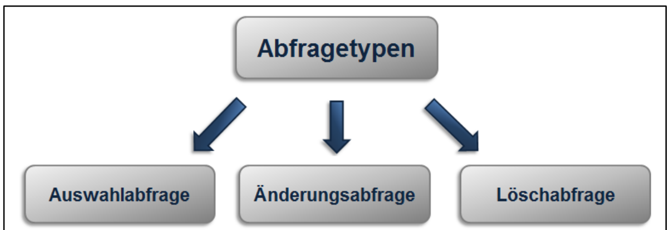
Abb. 177: Abfragetypen
